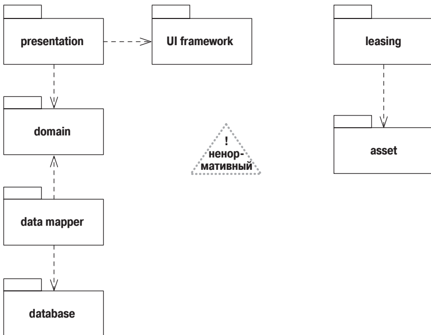
Рис. 7.3. Разделение рис. 7.2 на два аспекта
