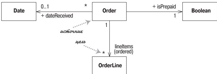
Рис. 3.3. Представление свойств заказа в виде ассоциаций
