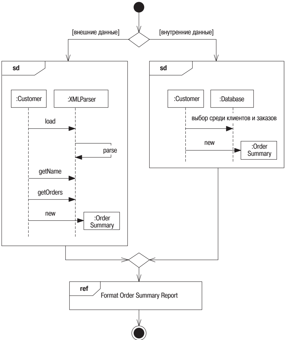
Рис. 16.1. Диаграмма обзора взаимодействий
