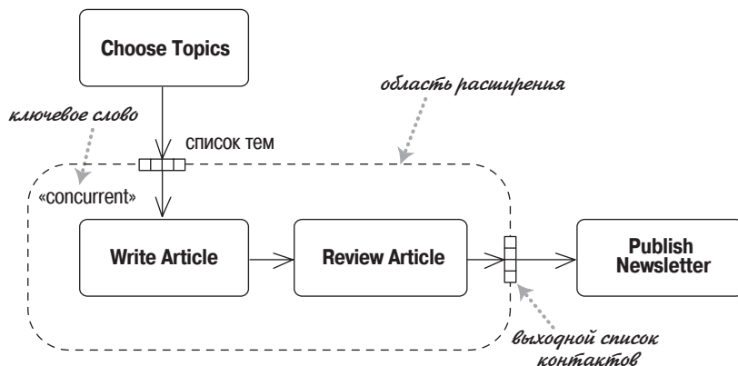
Рис. 11.9. Область расширения
