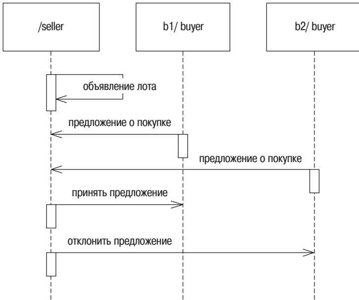
Рис. 15.2. Диаграмма последовательности для аукционной кооперации
