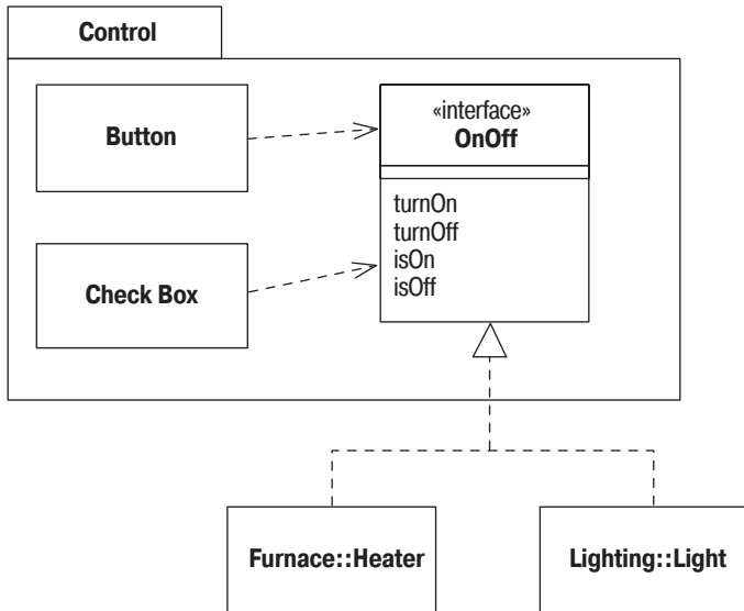
Рис. 7.5. Определение затребованного интерфейса в клиентском пакете
