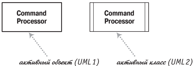
Рис. 5.21. Активный класс
