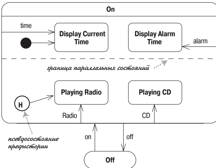
Рис. 10.5. Параллельные состояния
