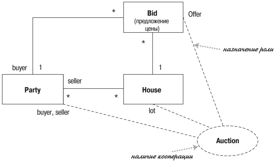
Рис. 15.3. Наличие кооперации
