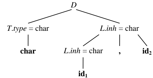
Рис. 2. Аннотированное дерево разбора строки char id 1 , id 2
