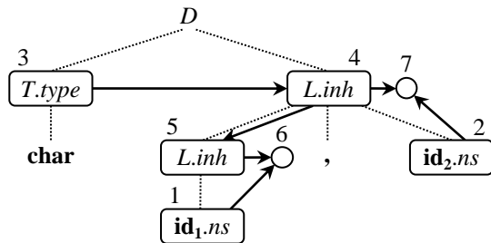
Рис. 3. Граф зависимостей для дерева разбора на рис. 2
