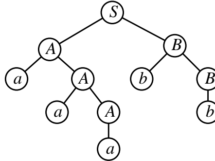
Рис. 1.2. Дерево разбора строки aaabb
