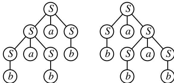
Рис. 1.3. Деревья разбора строки babab
